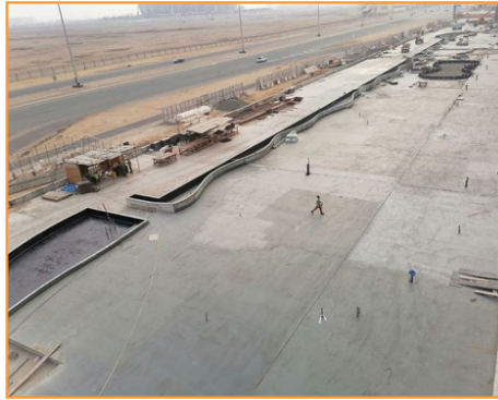
عزل البوليغارد Waterproofing of the boulevard
